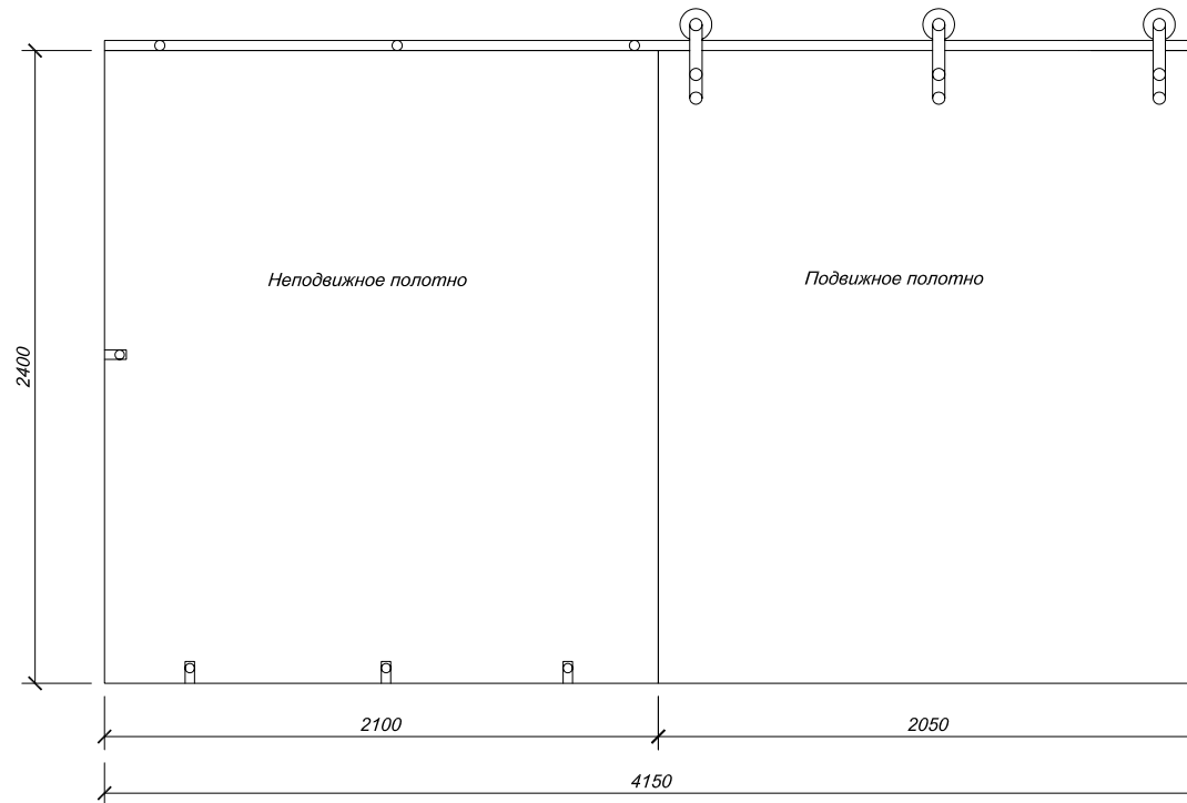
Раздвижная перегородка
