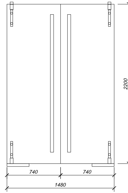
Проем Д-8
